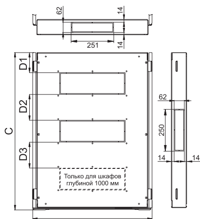
ВИД СНИЗУ
