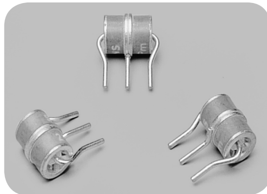
3-электродный разрядник без элемента термозащиты Fail-safe
