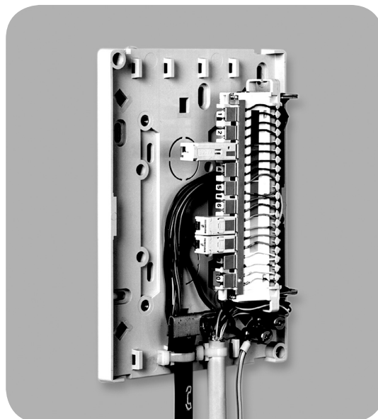
Минираспределитель ComGuard для установки штекеров защиты ComProtect
