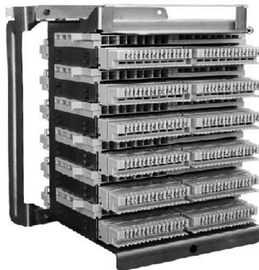
Универсальный блок главного кросса
