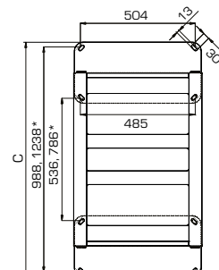
Вид снизу
